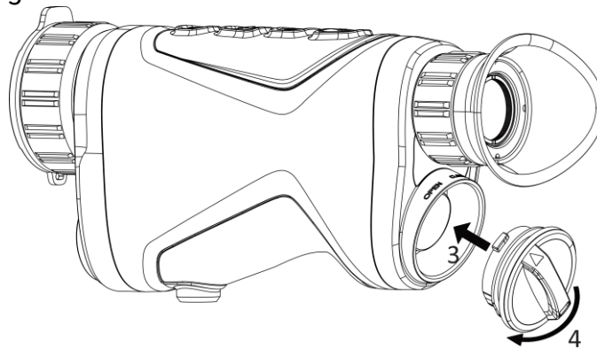
Abbildung 2-3 Abdeckung festziehen
